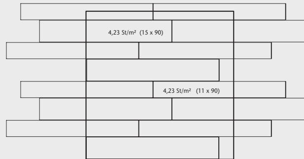
Verlegebeispiel 2
